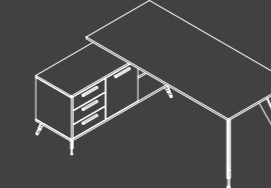
ETAJERLİ MASA DESK WITH ETAGERE 180X80X75 cm GZW180MS
